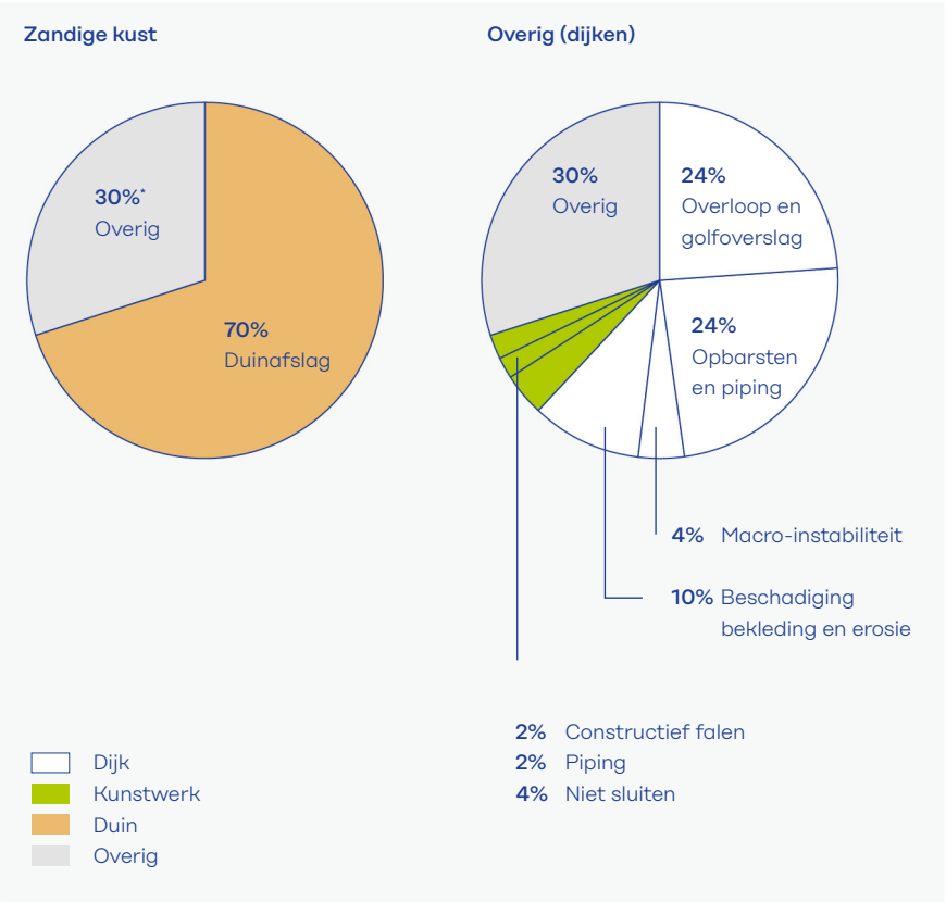
Figuur 5.7 De standaard faalkansbegroting bestaat uit maximaal toelaatbare faalkansen als percentages van de maximaal toelaatbare overstromingskans. Deze begroting is gehanteerd in het WBI2017 bij de gedetailleerde beoordeling. Afwijken van deze standaard faalkansbegroting is mogelijk zo lang het totaal 100% blijft.
