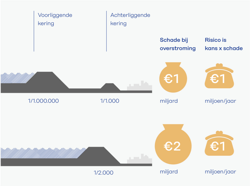
Figuur 4.13 Twee oplossingen, met en zonder voorliggende kering, die hetzelfde risico opleveren. Zonder voorliggende kering is de schade groter omdat er meer water binnenkomt.
