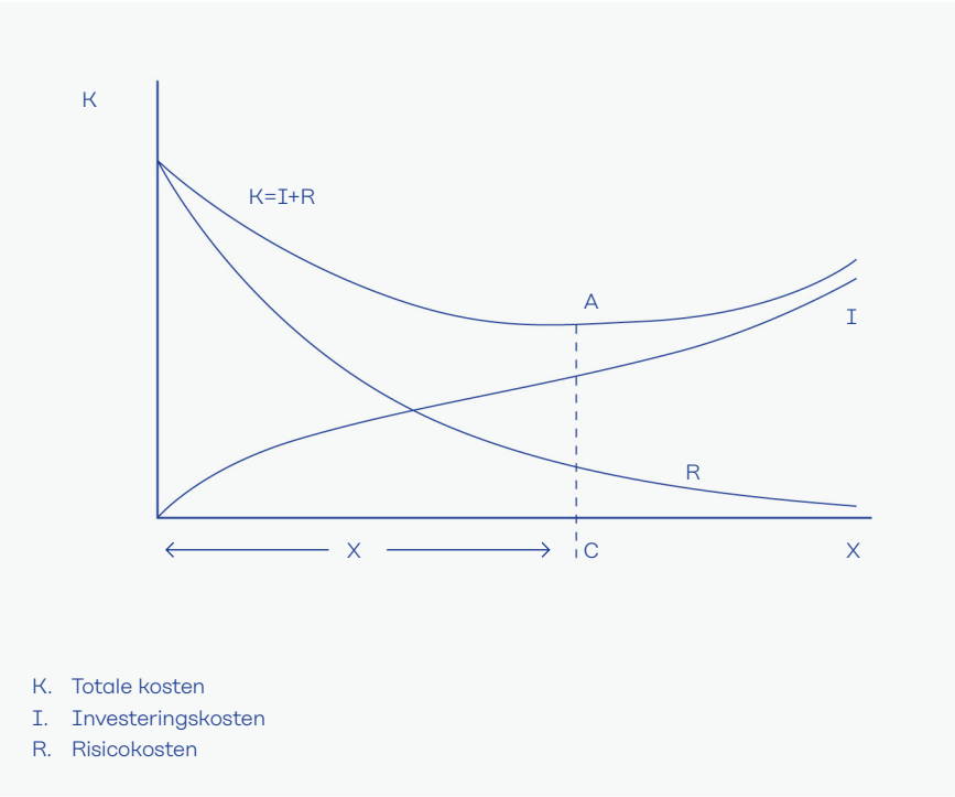
Figuur 4.8 Het basis-principe van een economische optimalisatie. De totale kosten (K) zijn gelijk aan de investeringskosten (I) voor vergroting van de betrouwbaarheid (hier: dijkverhoging) plus de contante waarde van het risico (R). Het optimum ligt waar de totale kosten (I+R) minimaal zijn.
