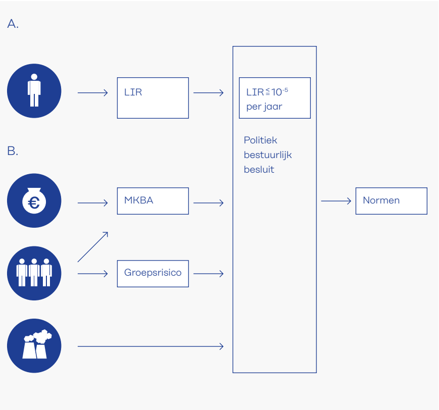
Figuur 4.2 De principes die ten grondslag liggen aan de overstromingskansnormen voor de primaire waterkeringen.
