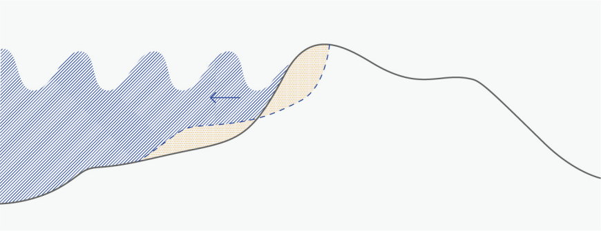
Figuur 5.2 geeft het faalmechanisme weer bij duinen, duinafslag. Golven leiden daarbij tot erosie van het buitentalud waardoor delen van het duin onder water verdwijnen en op het strand of vooroever worden afgezet. Als het duin te ver erodeert breekt het duin door. Het kan dan het buitenwater niet langer keren met een overstroming van het achterland als onontkoombaar resultaat.
