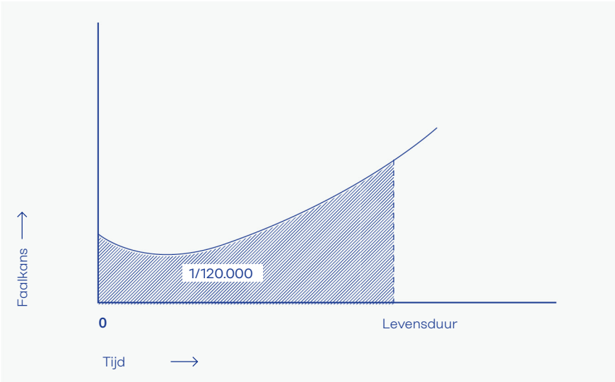
Figuur 6.3 Illustratie van een ontwerp op basis van gevolgklasse CC3 van de Eurocode: de kans op falen in de levensduur is gelijk aan 1/120.000 ( \beta=4,3 ).
