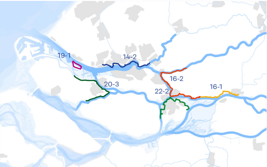
Figuur 4.12 De zes trajecten in het zuidwesten van Nederland waar bij de normstelling rekening is gehouden met het grote aantal slachtoffers dat hier zou kunnen vallen.
