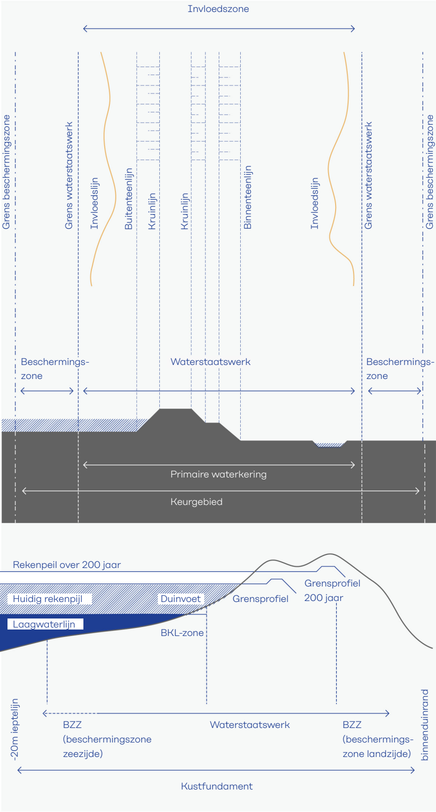
Figuur 7.3 Voorbeelden van keurzones van waterschappen.
