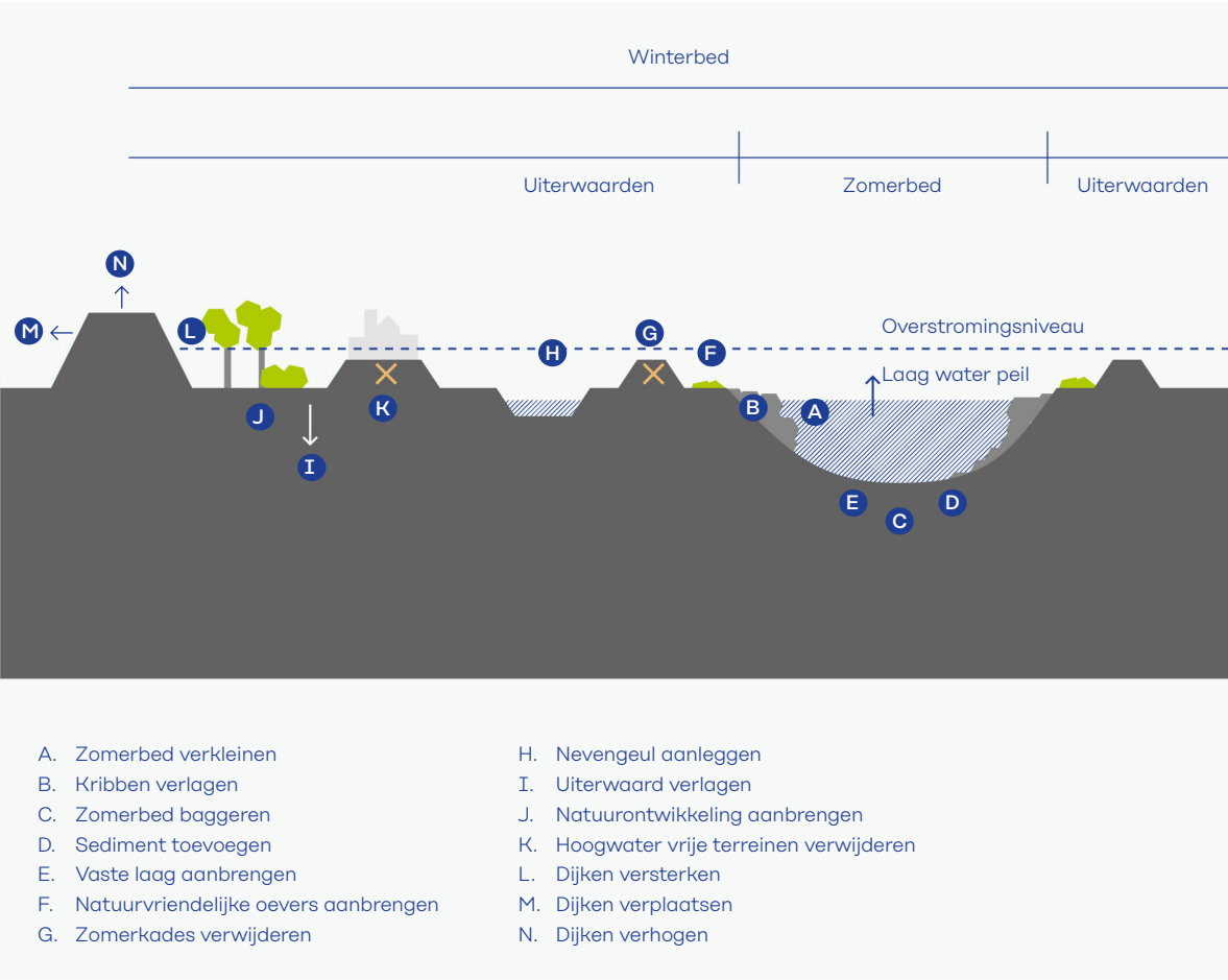
Figuur 6.4 Mogelijke maatregelen in het dwarsprofiel van de rivier.
