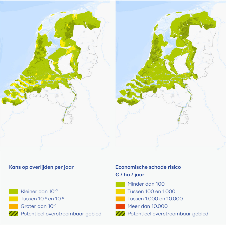
Figuur 4.4 Het lokaal individueel risico en het economische schade als alle keringen voldoen aan de eisen in de Waterwet.
