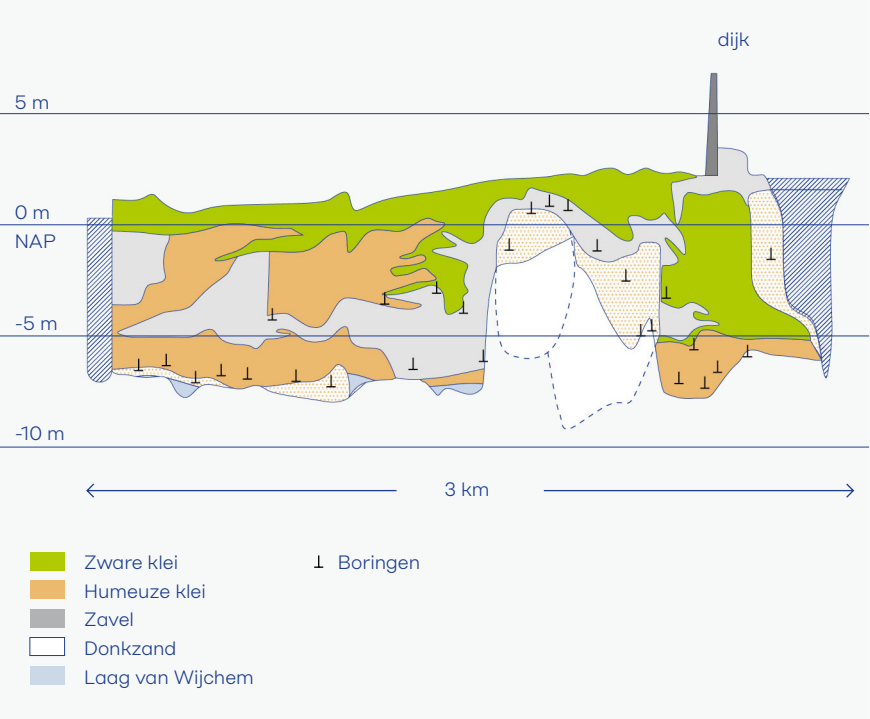
Figuur 3.2 Een overzicht van de laagopbouw volgens boringen en sonderingen. Tussen deze boringen en sonderingen is het onzeker hoe de ondergrond is opgebouwd.
