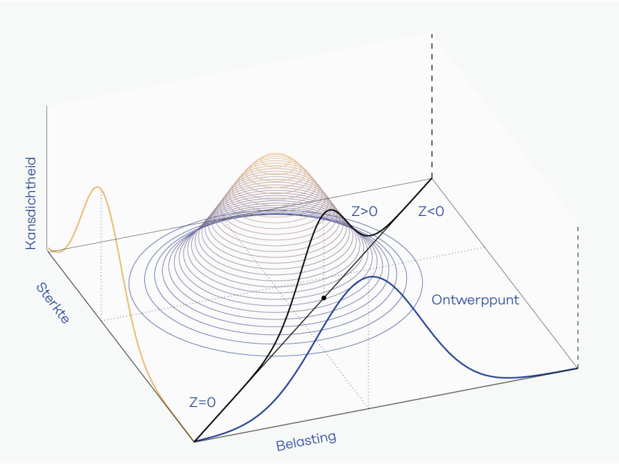
Figuur 5.8 De faalkans en de gezamenlijke kansverdeling van de sterkte en de belasting.
